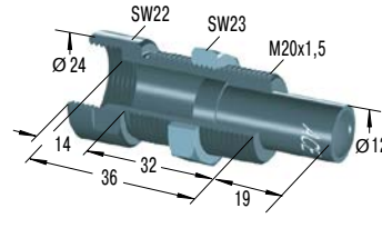
BV20SC *€ 50,62 Bolzenvorlagerung
