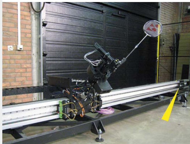
Unterschiedliche Dämpfer bremsen schnelle Bewegungen eines Badminton-Roboters
