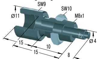
BV8 *€ 30,39 Bolzenvorlagerung
