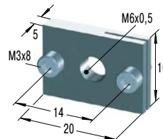
RF6 *€ 12,43 Rechteckflansch
