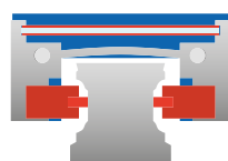
Elemento di bloccaggio sfiatato
