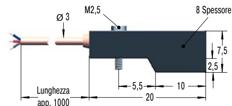
250-3 PNP Schema sensore PNP
