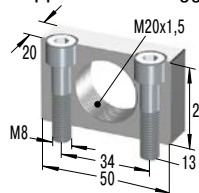
MB20SC2-V4A Supporto di montaggio
